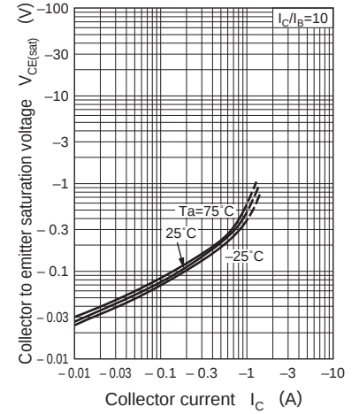
V_{CE(sat)} - I_C
