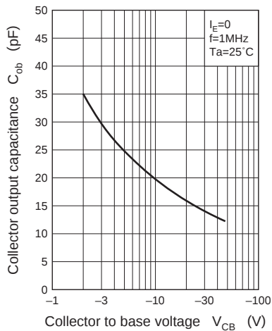
C_{ob} - V_{CB}
