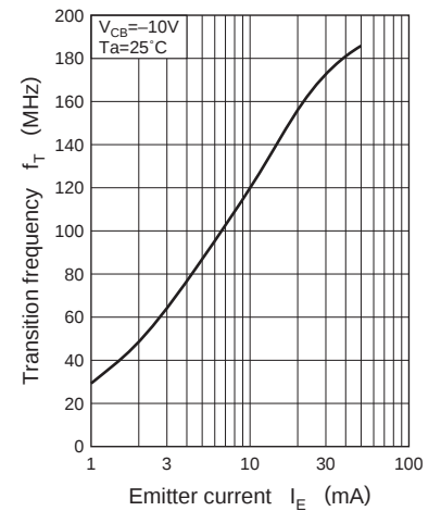
f_T - I_E
